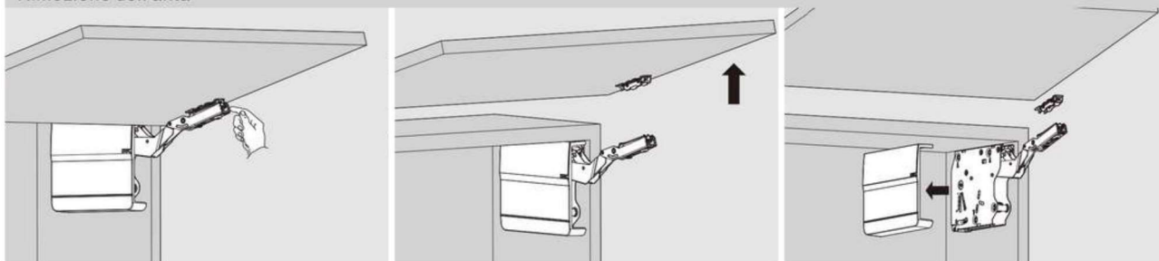
Rimozione dell'anta
